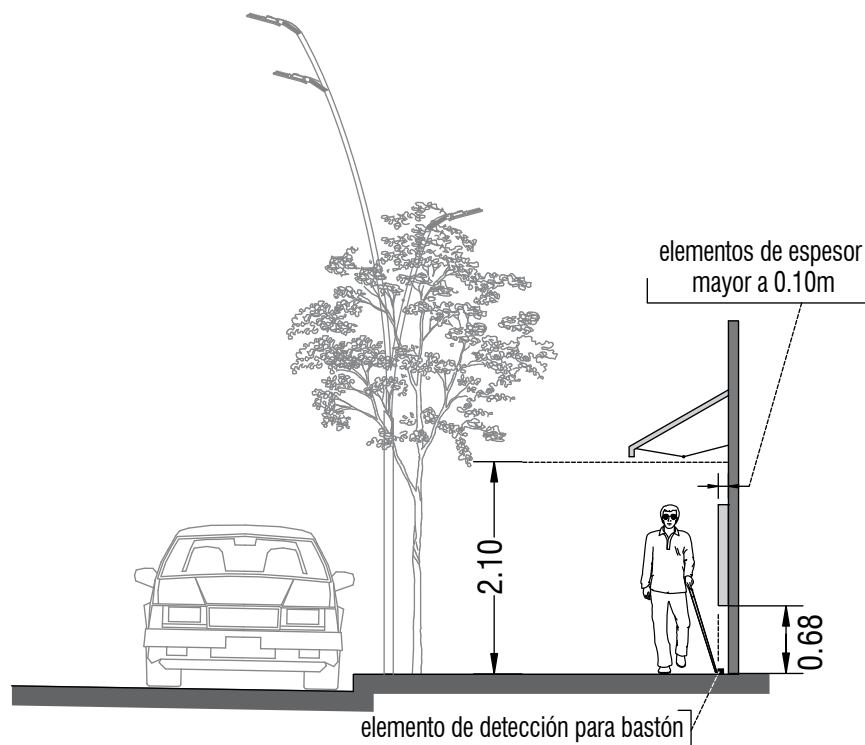
Elemento montado en muro
