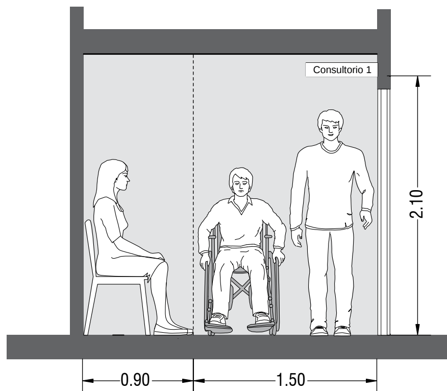
Medidas mínimas en circulaciones interiores
