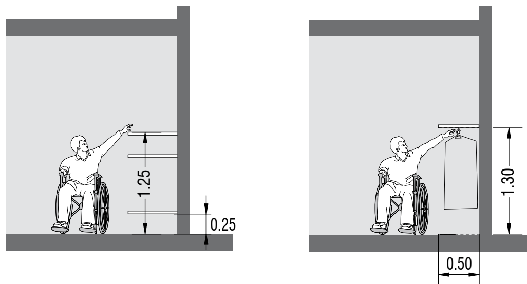
Dimensiones mínimas en dormitorios
