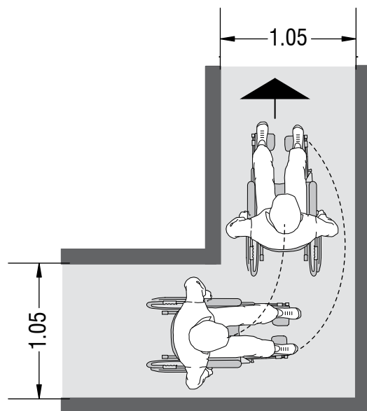
PASILLO ANCHO CONTINUO
