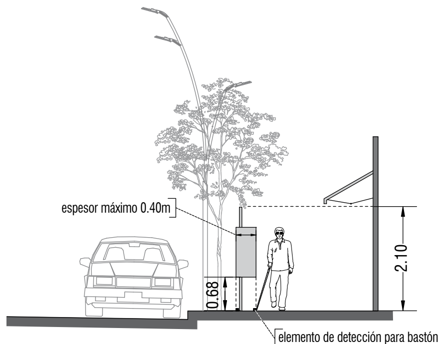
Elemento montado en un poste
