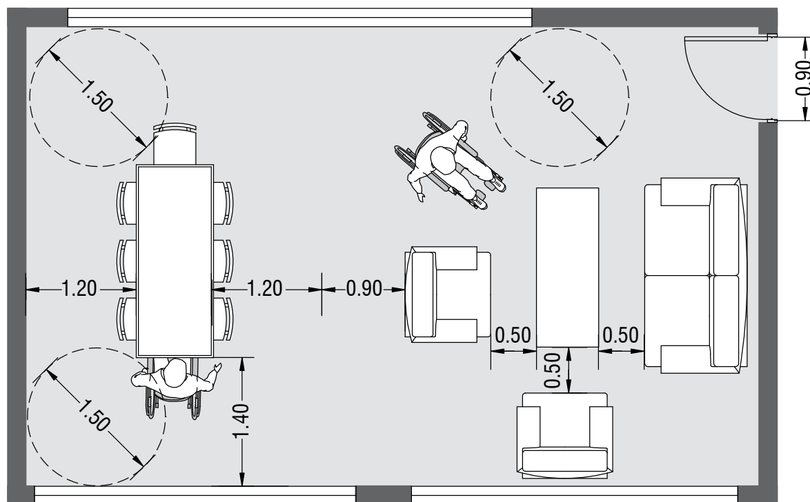
Estar-comedor: distancias mínimas en la disposición de mobiliario
