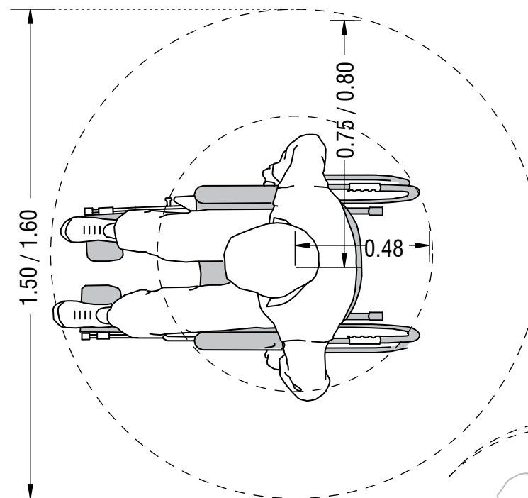
Vista superior (Planta)
